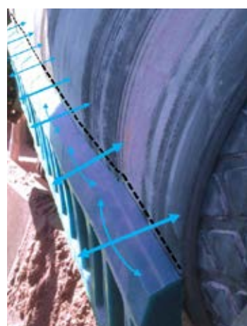
Les multi-lames du RacloFlex Z 2 épousent la forme de la bande et s'adaptent parfaitement
